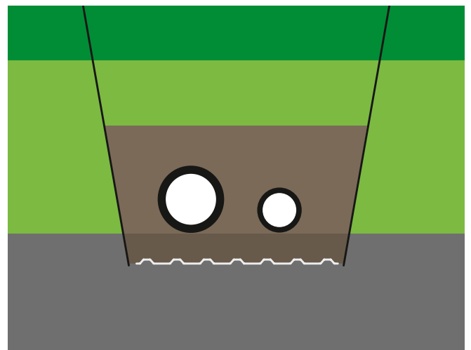
Poikkileikkaus kaivannosta
